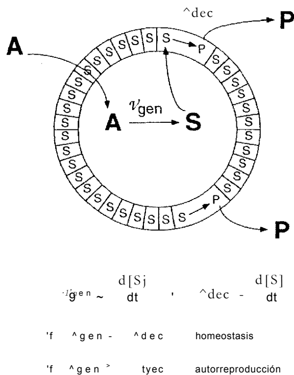
Figura 3: Esquema de la unidad autopoietica más sencilla posible. En este caso, en contradicción con la Figura 1 del extraterrestre, la barrera es una estructura físicamente especificada, es decir, es una membrana semipermeable o barrera. La figura 3 puede considerarse como una sobresimplificación de la conducta celular ilustrada en la Figura 2.
