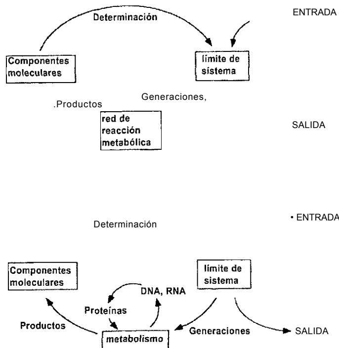
Figura 4: La circularidad del sí mismo en la organización autopoietica: En sus relaciones operacionales, los componentes moleculares determinan una red dinámicamente organizada y enlazada de transformación (metabolismo), que produce los componentes moleculares de la membrana, lo que, a su vez permite la operación de la red, y así sucesivamente. En nuestro mundo biológico, todo el sistema de reacciones está regulado por los ácidos nucleicos, como aparece graficado en la figura 4b. Tal como se señaló en el texto, la figura 4a representa el patrón más general, válido también para una vida «no codificada» (en la vida artificial o en los sistemas químicos sintéticos).
